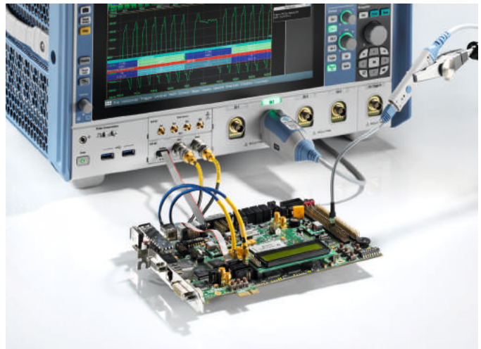
클록 신호로 내장형 임의 파형 발생기를 사용하여 LVDS 신호를 측정하며 8비트 패턴 발생기를 사용하여 제품에 대한 프로그래밍 및 제어
