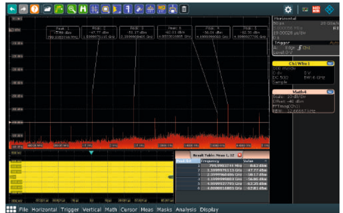
자동 피크 리스트 측정을 통한 고조파 및 상호 변조 분석
