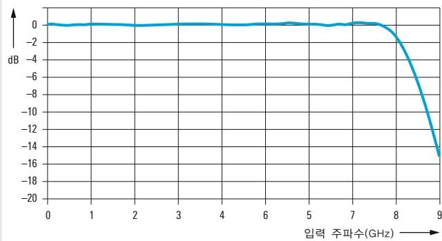
R&S®RTP084의 Flat frequency 응답성
