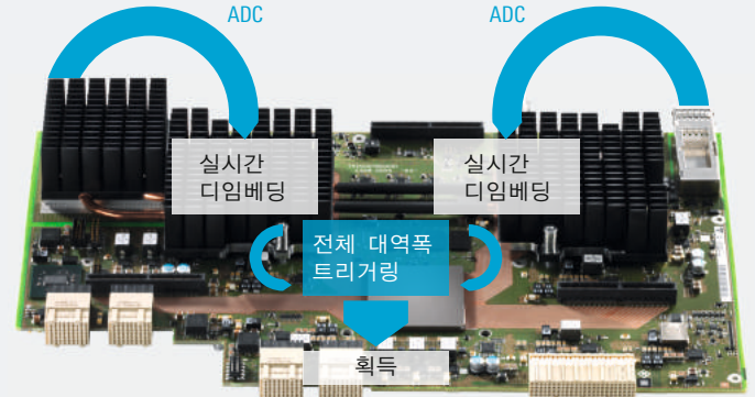
R&S®RTP 실시간 디임베딩 및 트리거 보드
