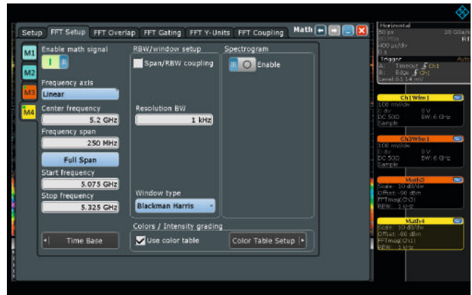
주파수 분석 설정은 일반적인 매개변수를 이용해 쉽게 설정할 수 있습니다.
