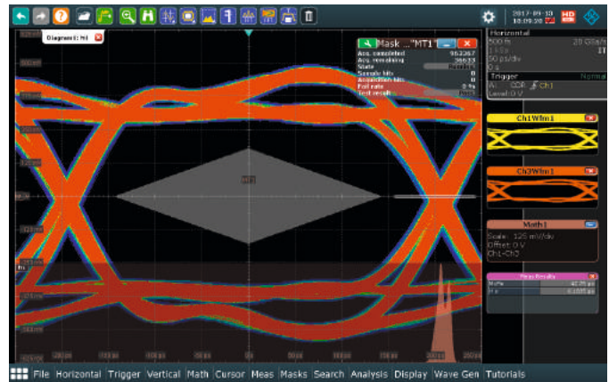
신속한 마스크 테스트 및 히스토그램
