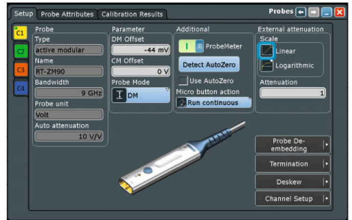
모듈식 프로브의 사용자 구성 매개변수가 적용된 설정 대화상자
